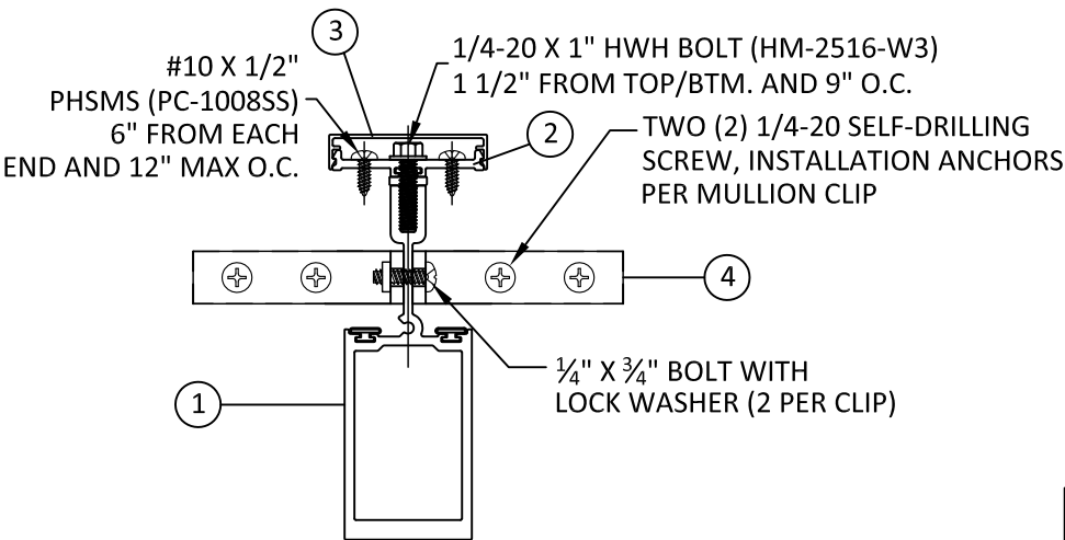
B 2 HORIZONTAL SECTION METAL STUD MULLION CLIP
